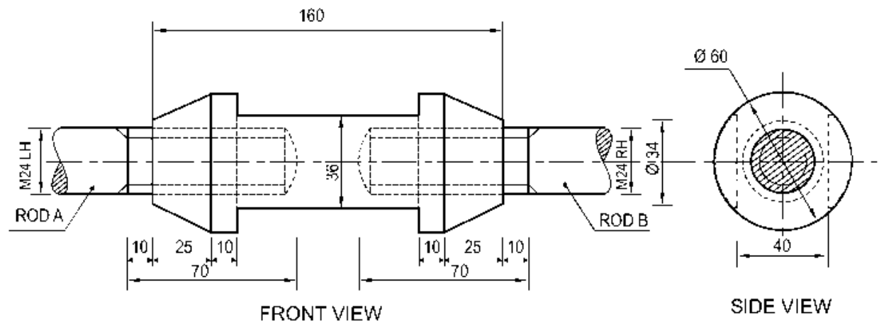
FIG 2 : TURNBUCKLE
