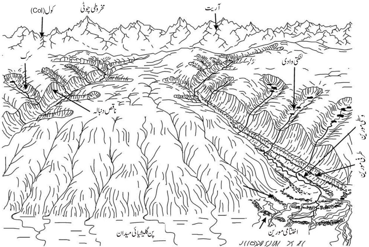
تصویر 7.12: کچھ گلیشیائی کٹاؤ اور جماؤی ہیئتیں (اپنسر، 1962 سے ماخوذ اور ترمیم شدہ)
