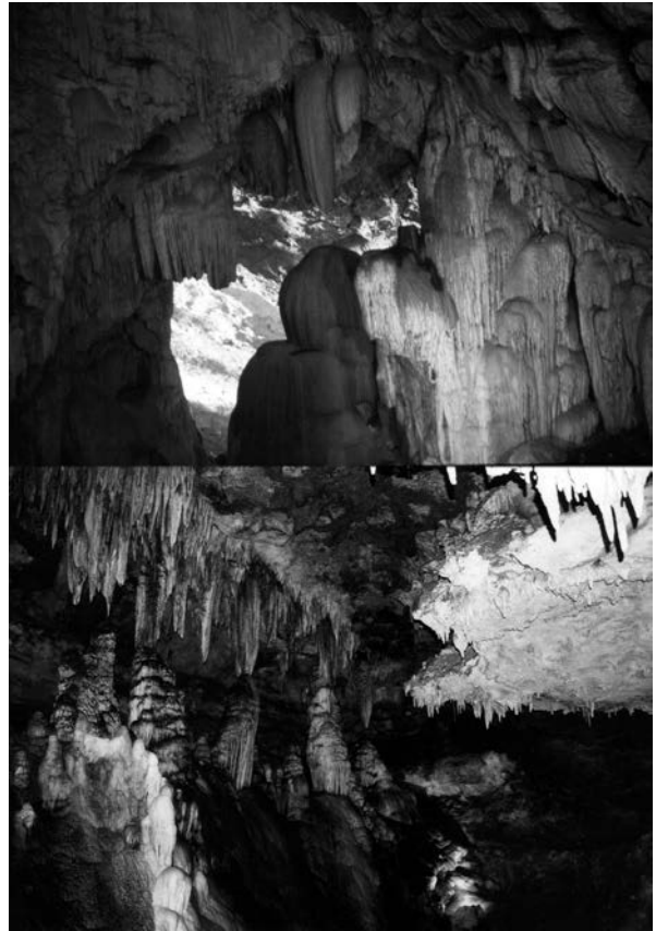
تصویر 7.10: ایک چونا پتھر غار میں اسٹیلک ٹائٹ اور اسٹیلک مائٹ
