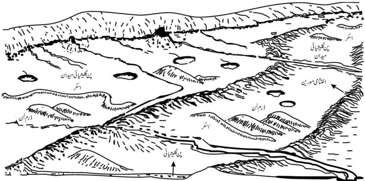
تصویر 7.13: مختلف جمادی ارضی ہیئتوں کے ساتھ گلشیائی زمینی منظر کا ایک سیریز خاکہ (اپنبر، 1962 سے ماخوذ اور ترمیم شدہ)
