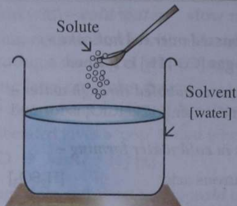
SOLUTE [Sodium chloride]
