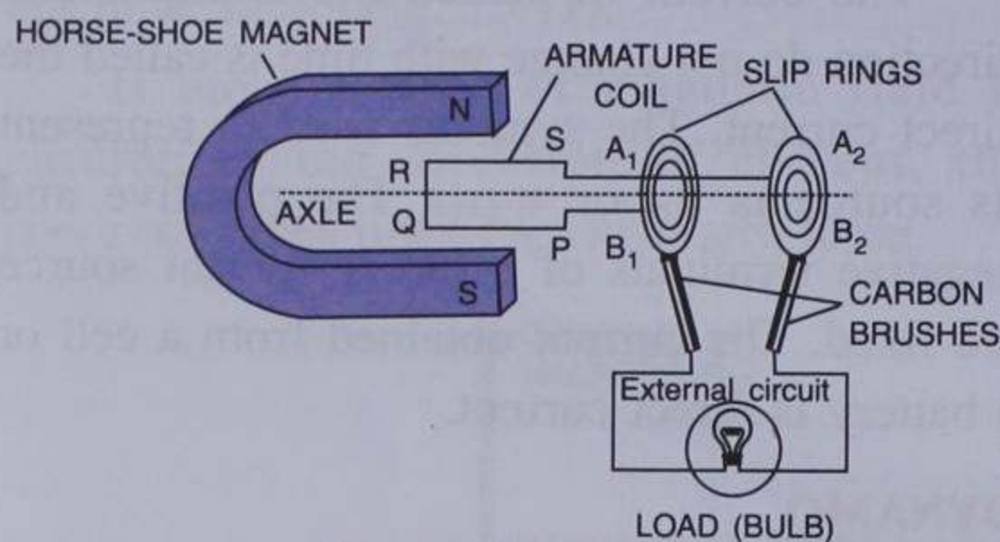
Fig. 13.13 Dynamo
