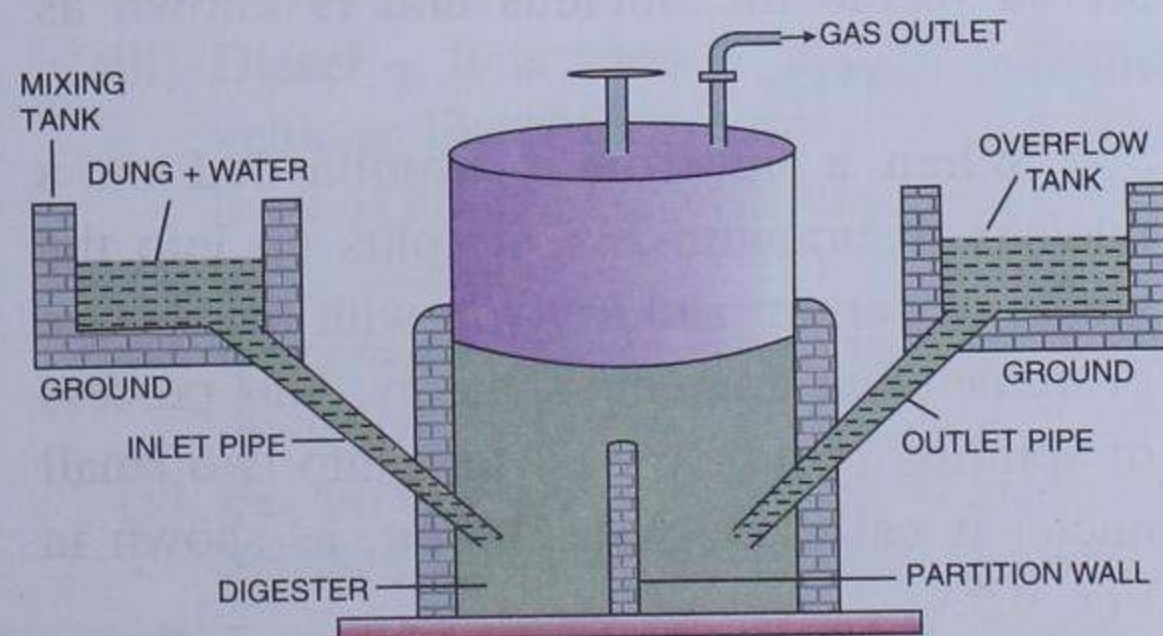
Fig. 9.4 : Biogas plant
