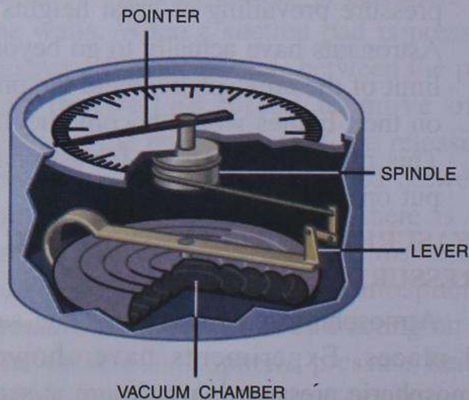
Fig. 7.14 Aneroid barometer
