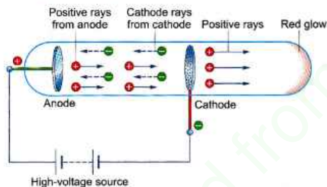
Fig. 4.5 Anode rays
