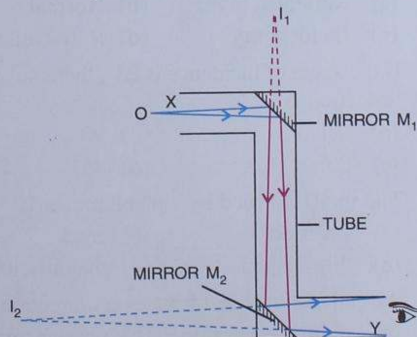
Fig. 6.11 Periscope
