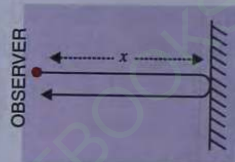
Fig. 3.19 Echo
