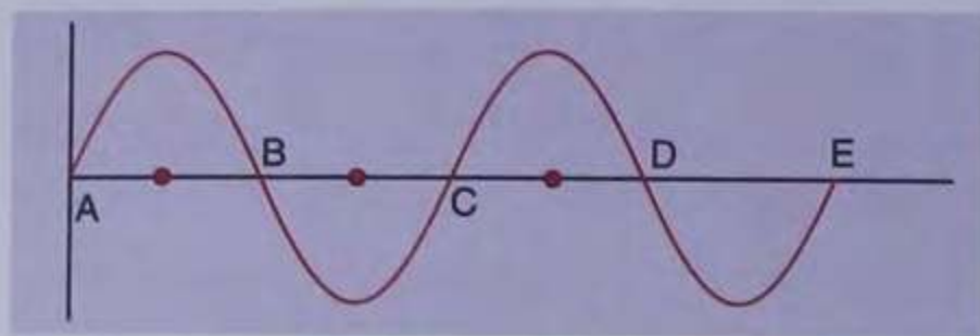
Fig. 3.4 A wave
