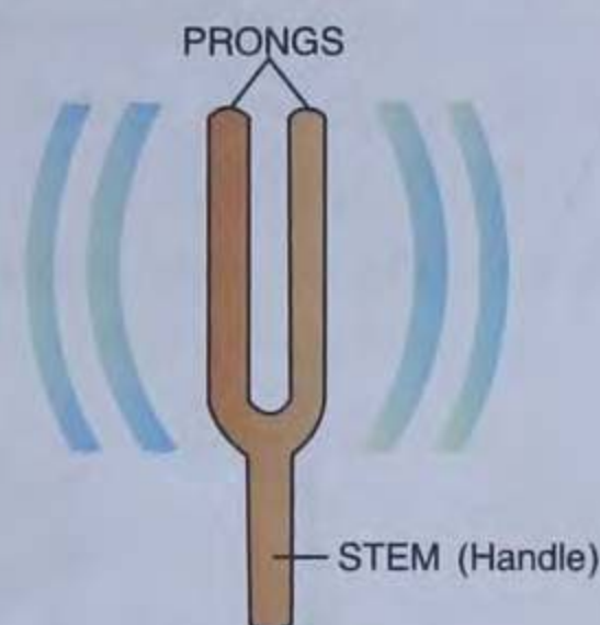
Fig. 3.12 Tuning fork
