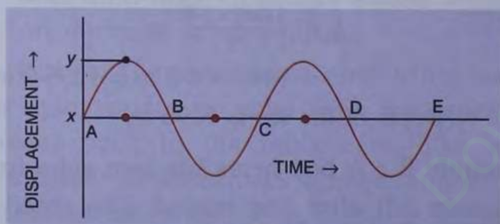
Fig. 3.21 A wave
