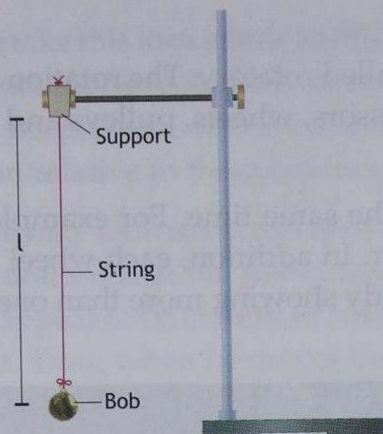
Fig. 2.4 Simple pendulum
