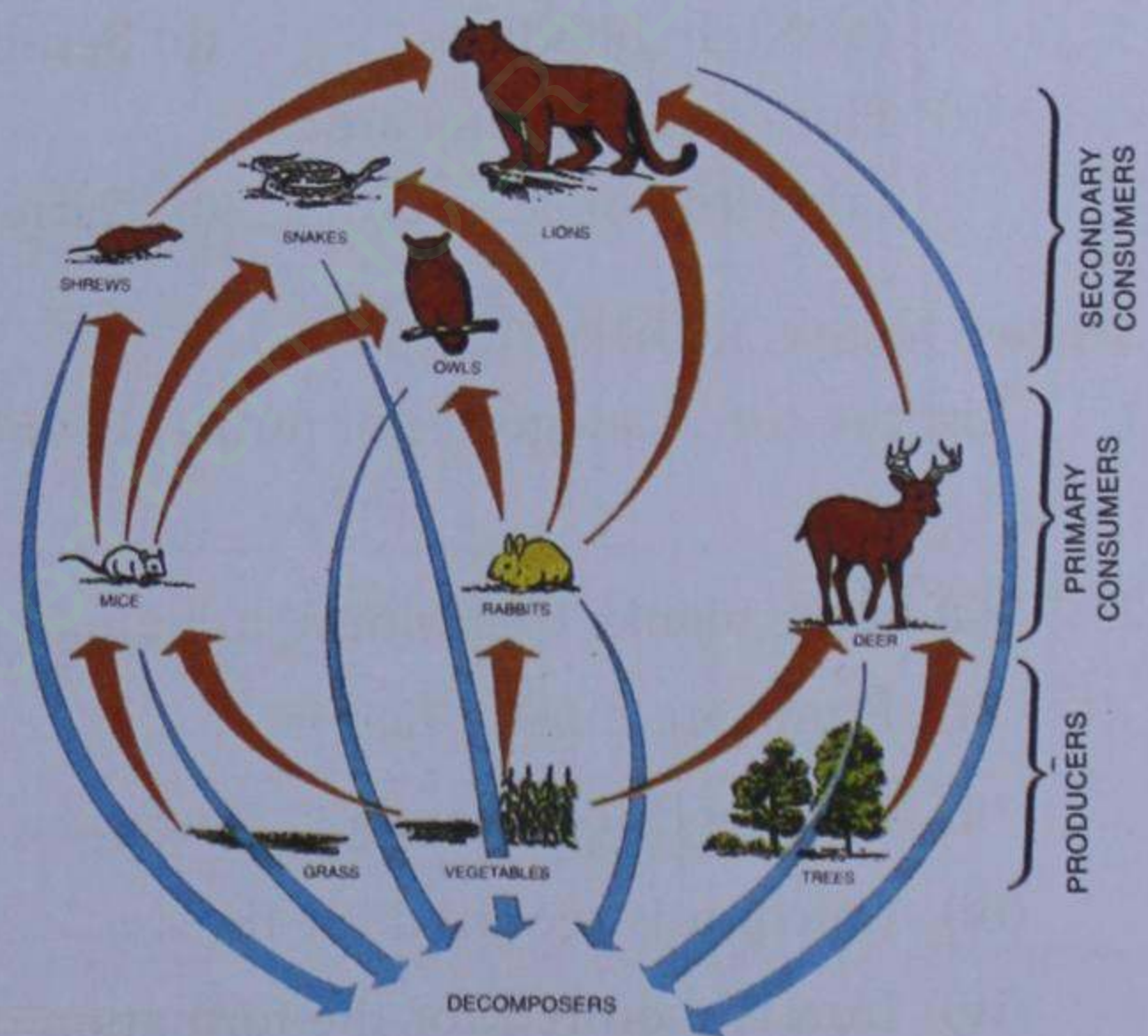
Fig. 4.9 Food web
