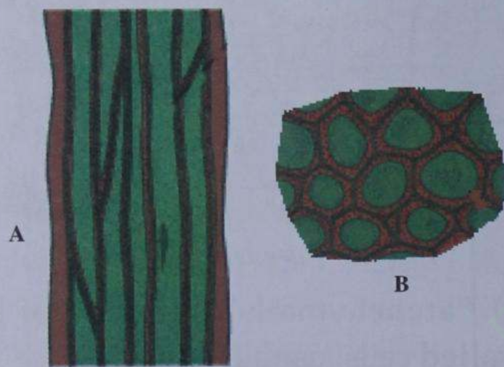
Fig. 2.8 Sclerenchyma
