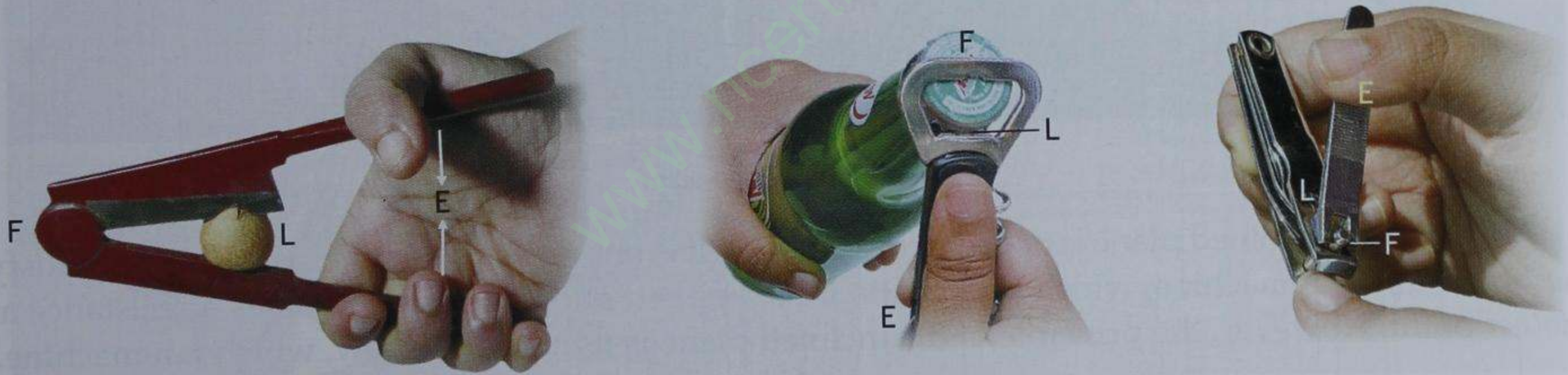
Fig. 5.9 Class-two levers
