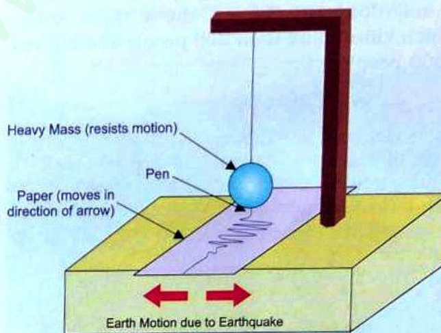
Fig. 8.4. Seismograph
