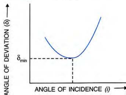
Fig. 4.24 i - \delta curve
