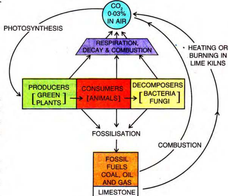
Fig. 6.10 : Carbon cycle
